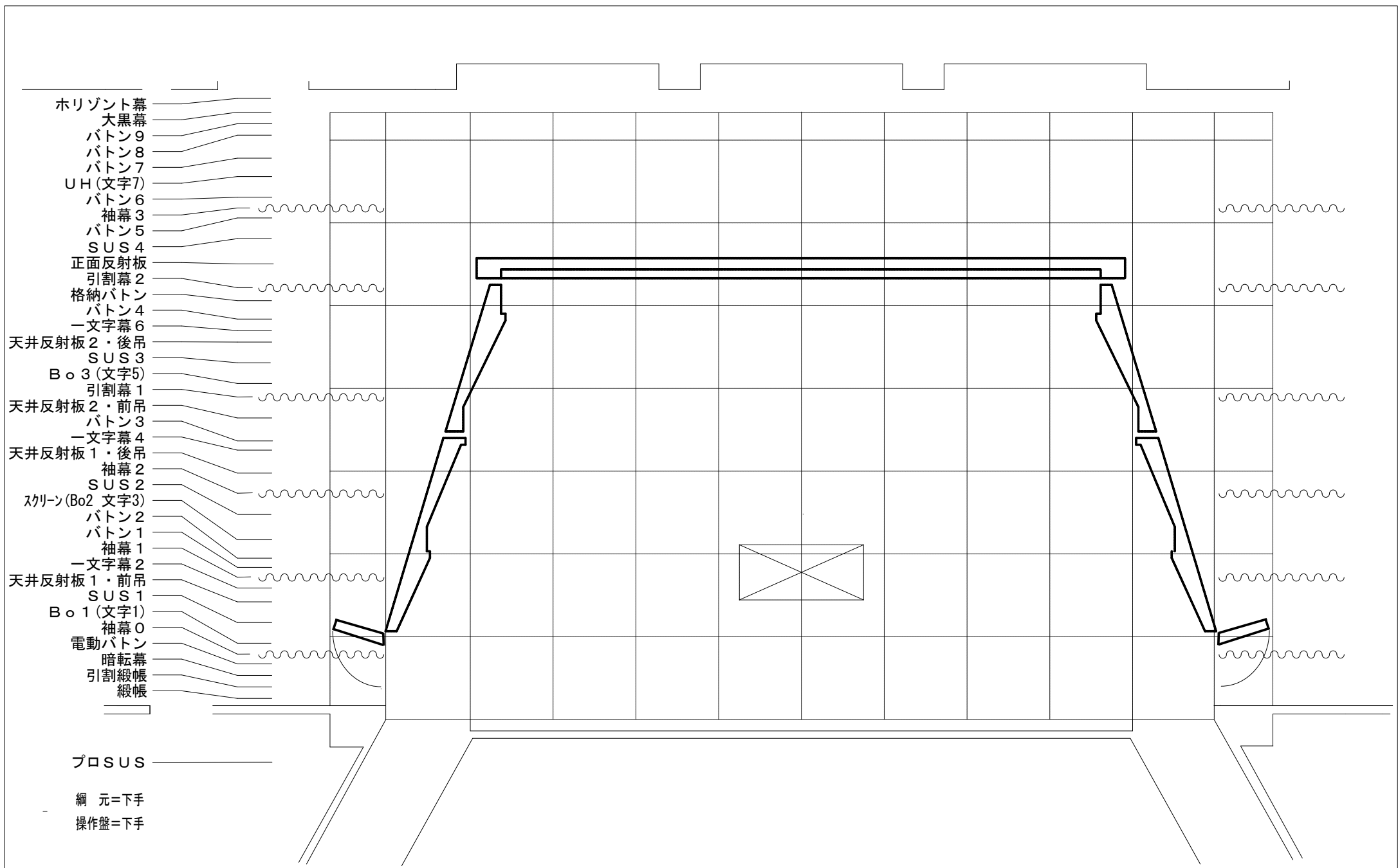
大町市文化会館 舞台仕込み図(反響板)
