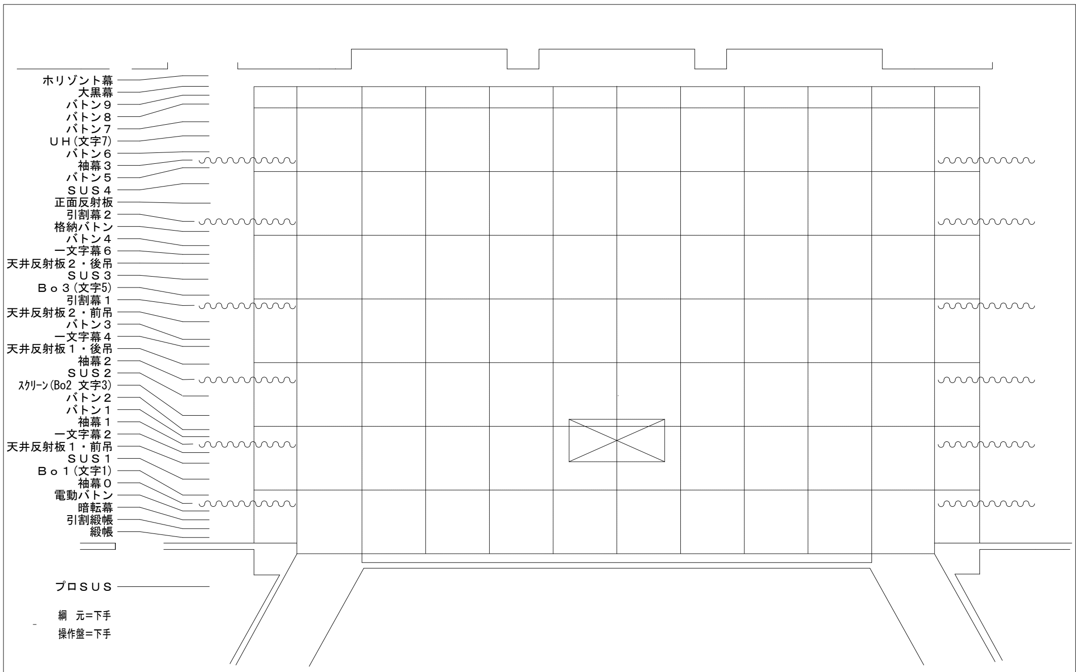
大町市文化会館 舞台仕込み図
