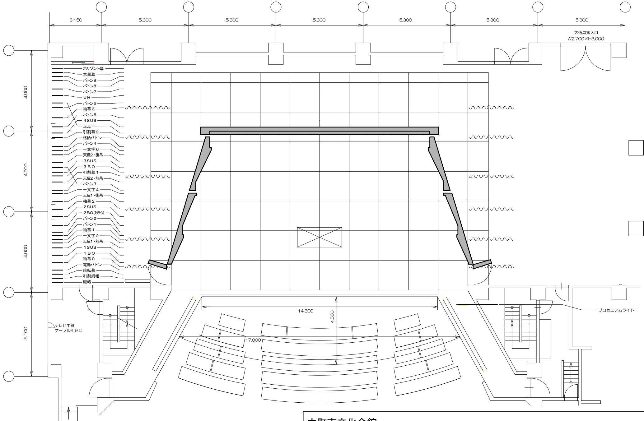
大町市文化会館 舞台平面図(反響板)
